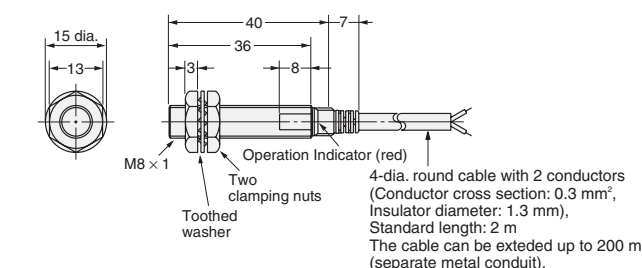
Fig. 8 : E2E-X3D□-N E2E-X2E□/F□
