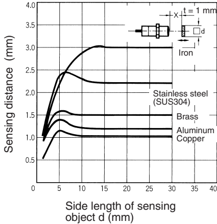
E2E-X4MD
