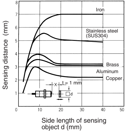
E2E-X8MD
