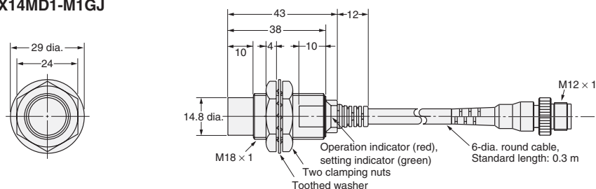
Fig. 33 : E2E-X14MD1-M1GJ
