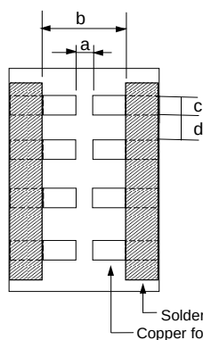
Fig. 3 (in:mm)
