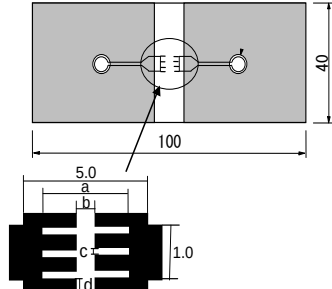
Fig. 1 (in:mm)
