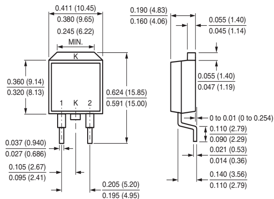
TO-263AB
