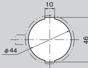
パネル穴明け寸法 Panel drilling dimensions
