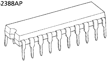
DIP20-P-300-2.54A
