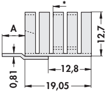
FK 237 SA 220... 21 K/W
