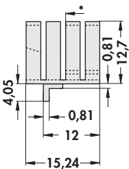
FK 242 SA 220 H 26 K/W
