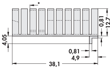
FK 240 SA 220 H 16 K/W
