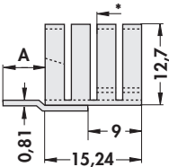
FK 242 SA 220... 26 K/W
