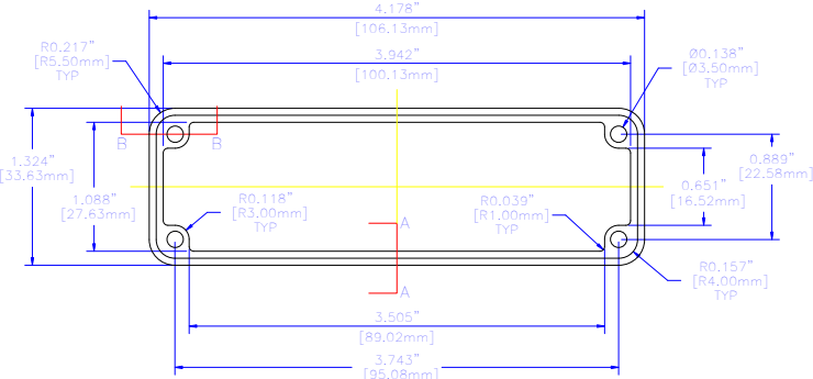
BEZEL
