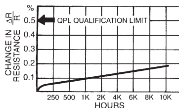
LIFE TEST
