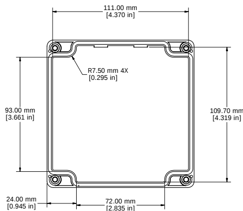
LID - INSIDE
