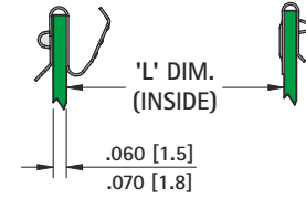
Fig. 1 Spring-Button
