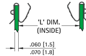
Fig. 2 Spring-Spring
