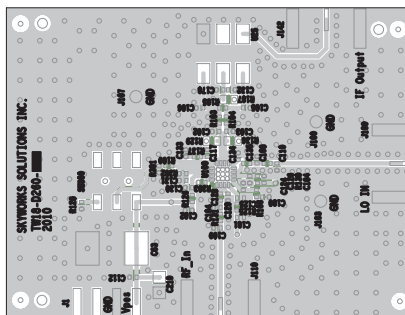
Layer 1: Top – Metal
