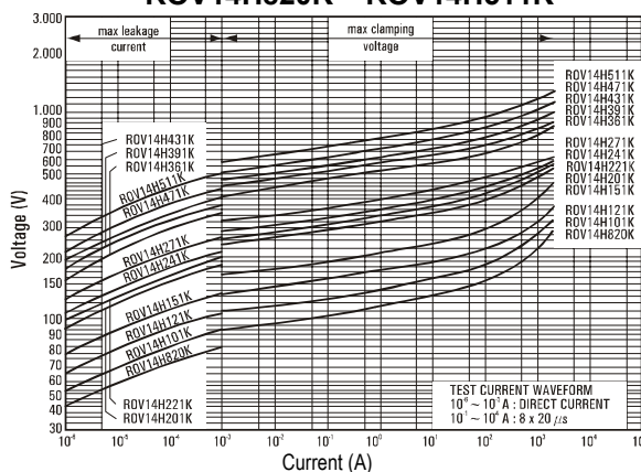
ROV14H820K – ROV14H511K
