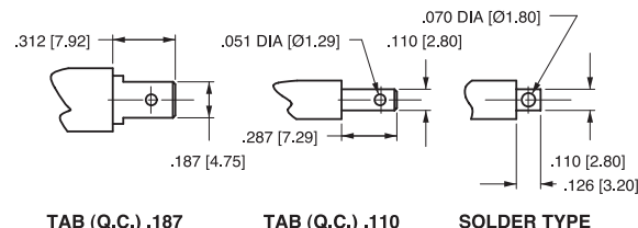
TAB (Q.C.) .187
