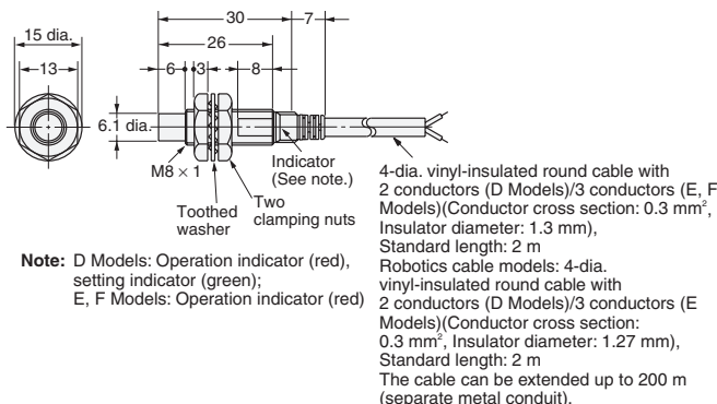
Fig. 8: E2E-X2MY
