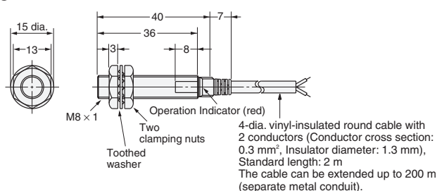
Fig. 9: E2E-X3D-N E2E-X2E/F
