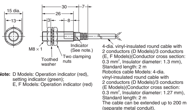
Fig. 7: E2E-X1R5Y
