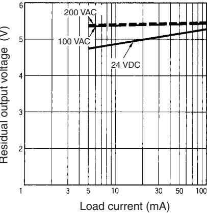
E2E-X□T1
