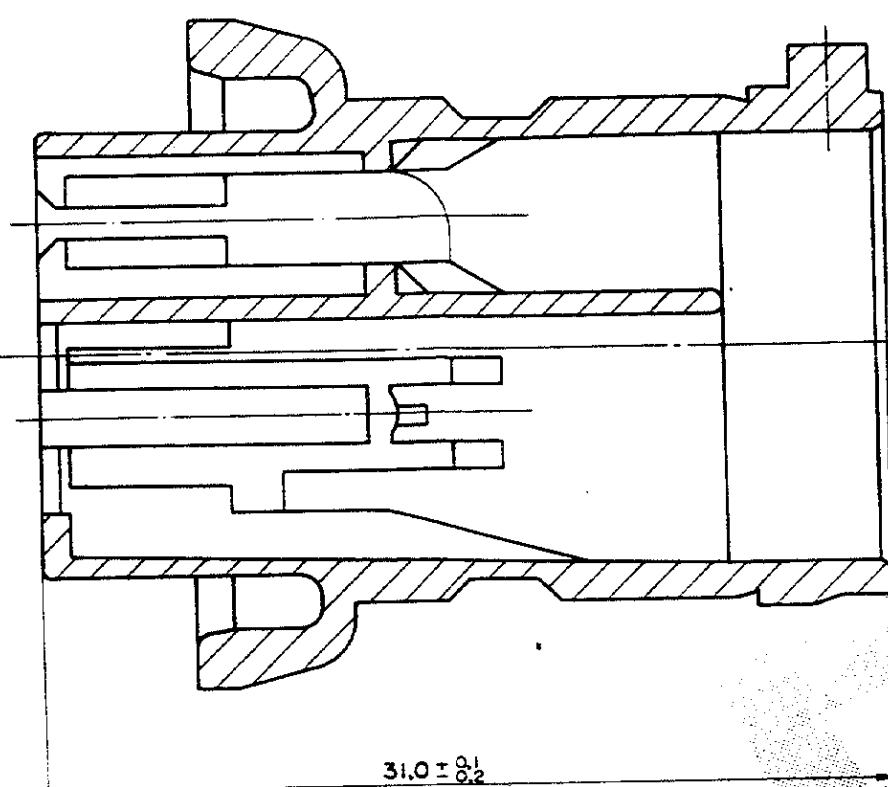
SECÇÃO AA
