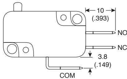
Quick connect terminal 187 series (D)
