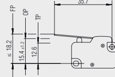
L02: gerader Hebel
