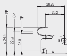
L31: Federhebel
