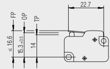
L01: gerader Hebel
