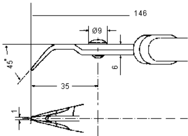
Dimensions : Millimetres
