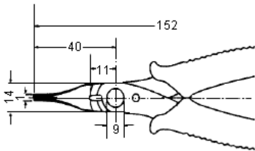
Dimensions : Millimetres
