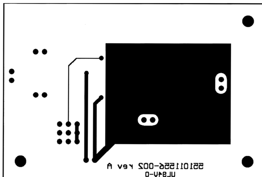
Figure 47. Bottom Layer
