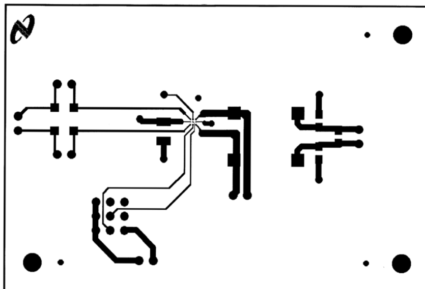
Figure 47. Bottom Layer
