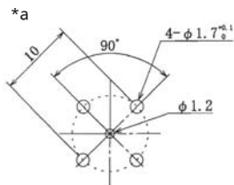
*a Leiterplattenlayout printed circuit board layout modèle de la carte imprimée
