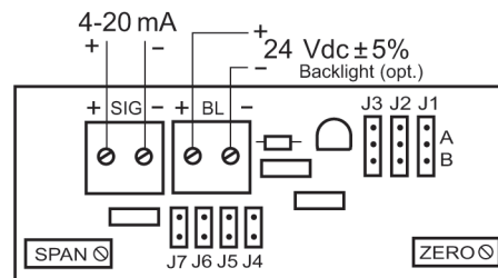
WIRING
