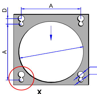
Lochbild 4 Steck-Schubmontage
