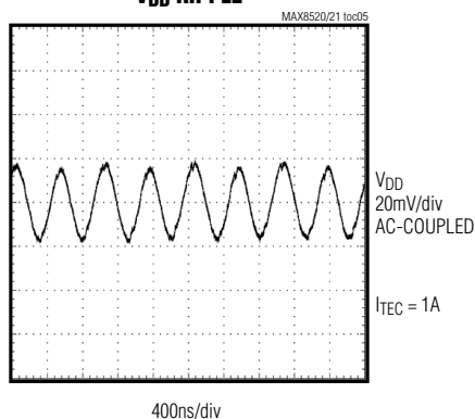
V_{DD} RIPPLE
