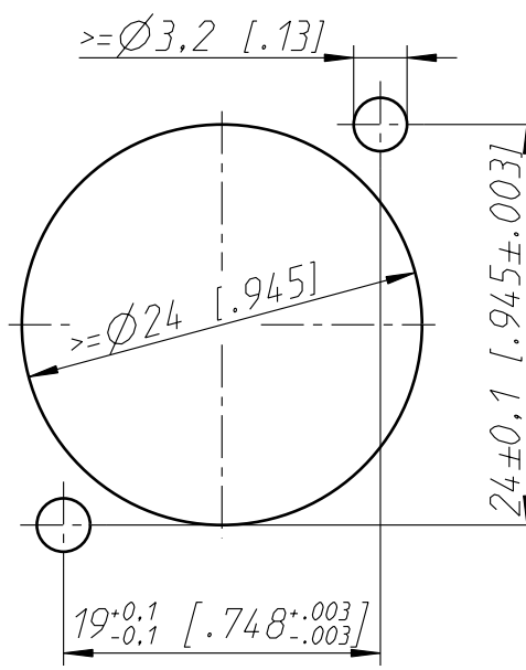
Frontplattenausschnitt (Rueckseite) Panel cut out (rear side)
