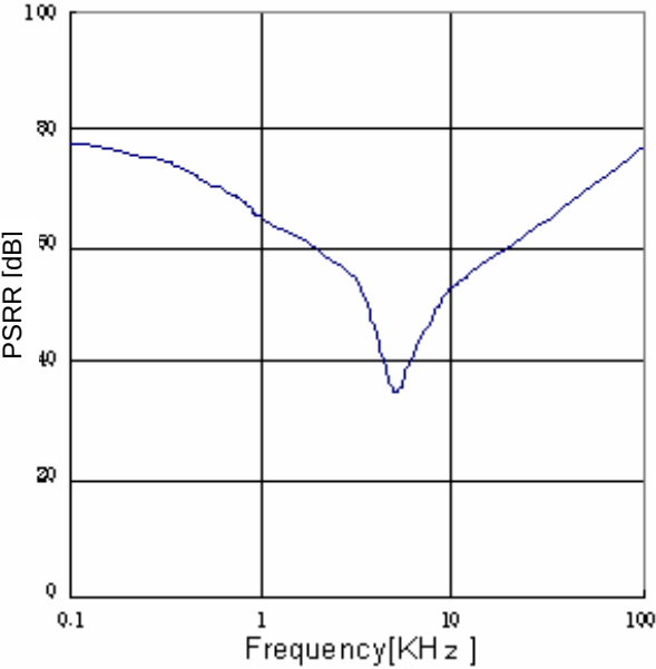
Fig.32 PSRR (Io=0mA)
