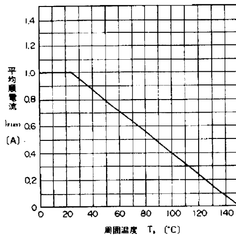
平均順電流—周囲温度特性 Current Derating ( I_{F(AV)}-T_a )
