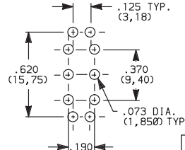
7201J1_BE2 DPDT
