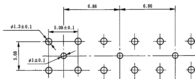
DM-CR-SSD backboard dimensions (JDAMB-3W3S)
