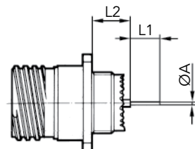
Receptacle type 0
