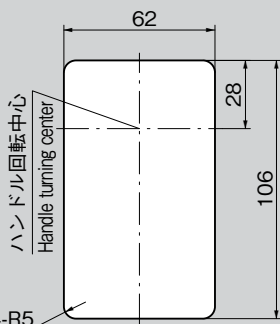
パネル穴明け寸法 Panel drilling dimensions
