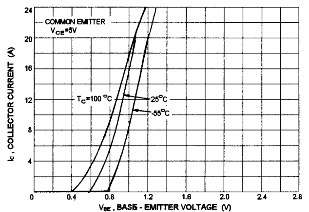
I_C - V_{BE}
