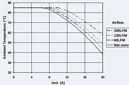
PT7715; V_{in} = 5V
