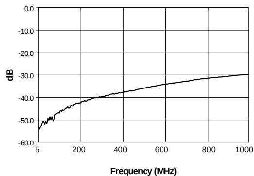
L-I Isolation
