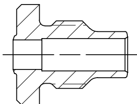
125123 ANVIL INSERT (-08)
