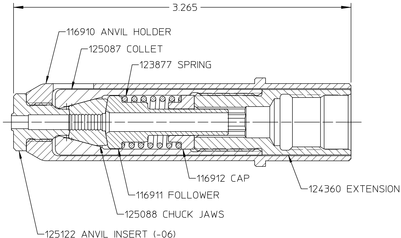
SECTION A-A
