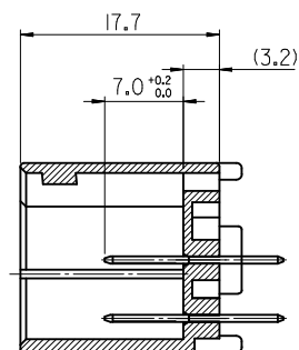
SECT.A-A
