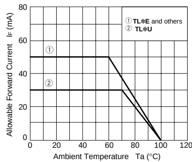
I_f - T_a
