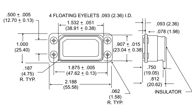
DPAF-34
