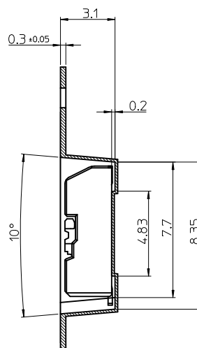
Section A-A
