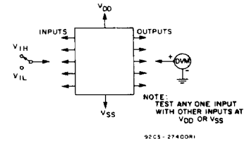
Fig. 16 - Input voltage test circuit.
