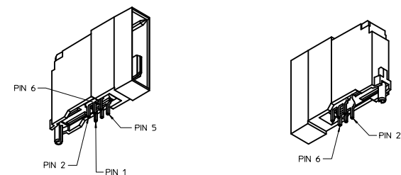
75561-1510 SHOWN (W/PEG)
