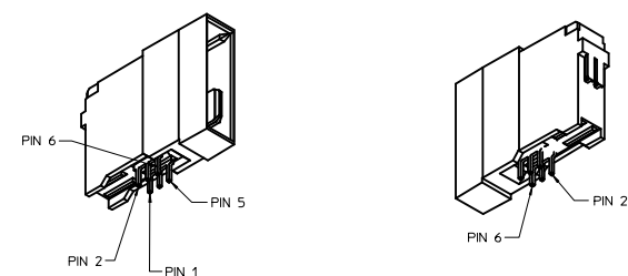
75561-5100 SHOWN (W/O PEG)
