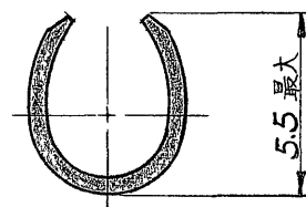
断面 C-C
