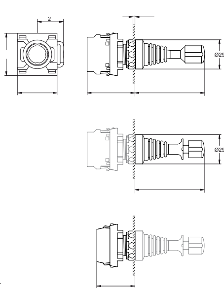
Joystick
