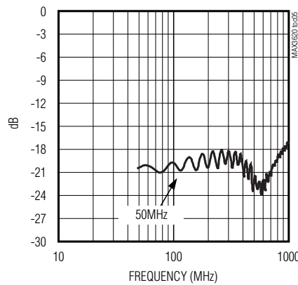
MAX3620A S11
