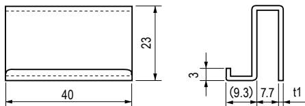
TL-134-3 受金具 Keeper
