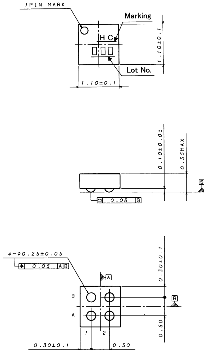
VCSP50L1 (UNIT:mm)
