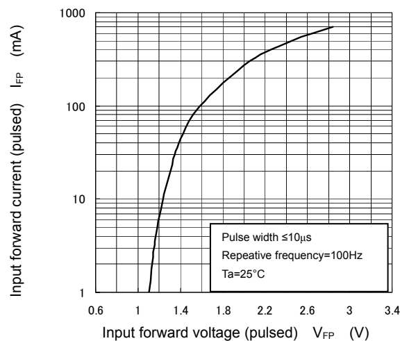
I_{FP} - V_{FP}
