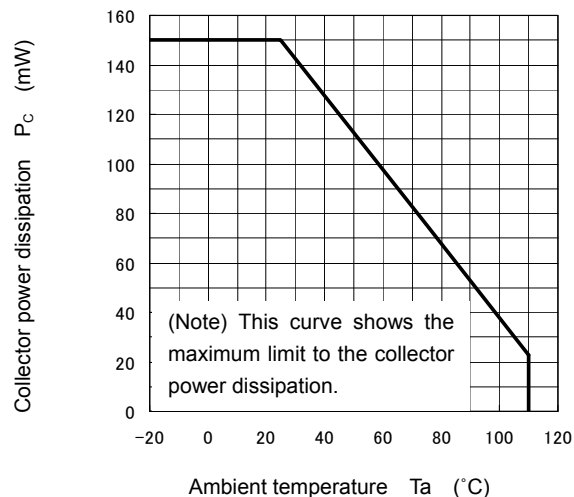
P_C - T_a
