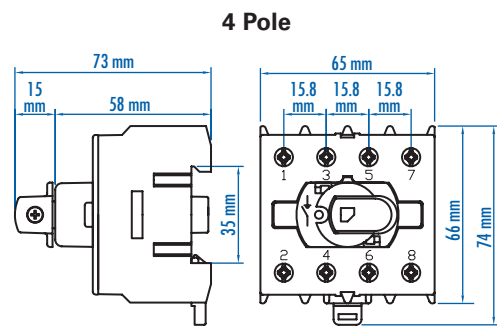
4 Pole
