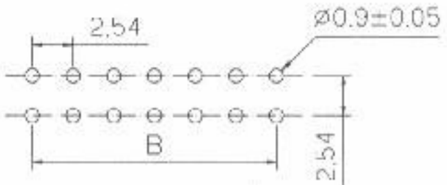
Double Row P.C.B. Layout
