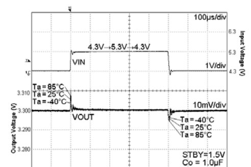
Fig. 178 VIN Response I_{out} = 10\text{mA}
