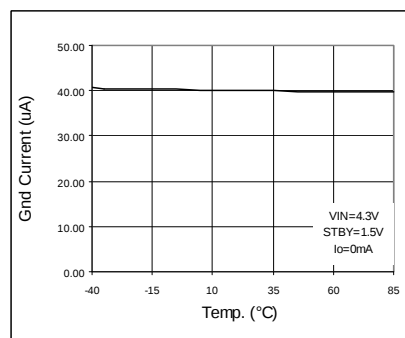
Fig. 160 IIGN vs Temp
