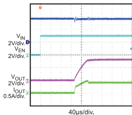
Enable On
